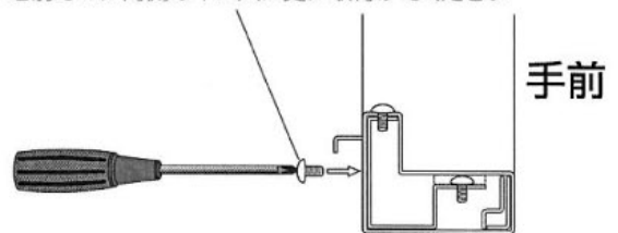
地前カマチを横から見た図
